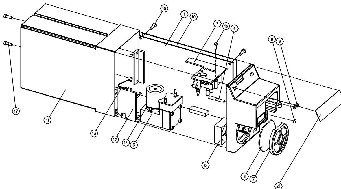
Figure 20 Exploded view, M-C rev.00, M-C0 rev.00, M-CAi0 rev.00, M-COV rev. 01, M-CAiOV rev.01, M-COVX rev.00
