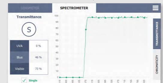
Pourcentage de transmission de la lumière visible, UV-A et lumière bleue
