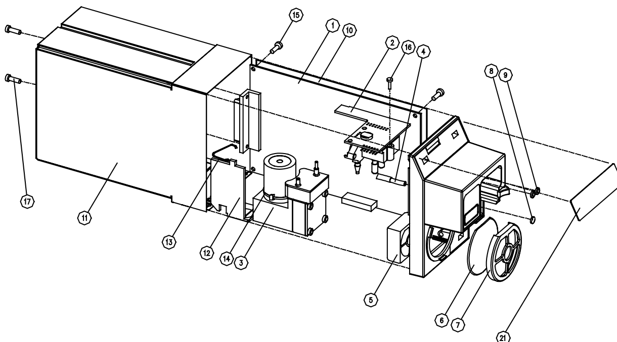
Figure 18 Exploded view, M-C rev.00, M-CO rev.00, M-CaiO rev.00, M-COV rev. 01, M-CaiOV rev.01, M-COVX rev.00
