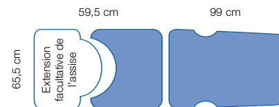
Longueur totale avec extension d'assise 186,5 cm
