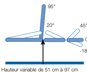
Modèles B & C avec option cyphose électrique
