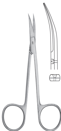
IRIS 012-271-090 9,0 cm / 3 1/2" 012-271-105 10,5 cm / 4 1/8" 012-271-115 11,5 cm / 4 1/2"
